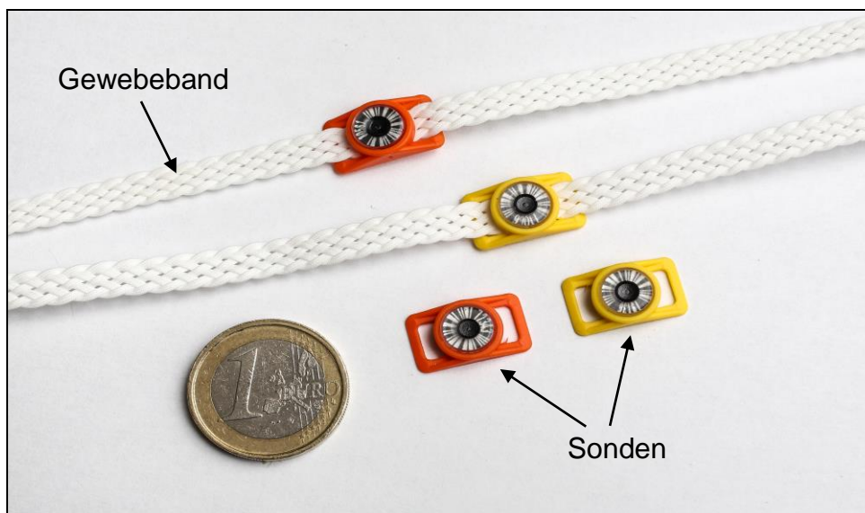
Bild 1: Sonden und Halterungen für Armband-Dosimeter
